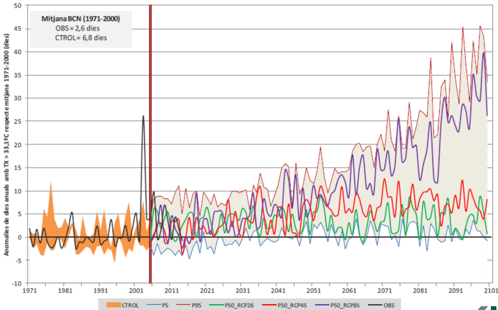
Evolució temporal projectada dels Dies anuals mitjans amb \text{TX} > 33,1^{\circ}\text{C} al T.M. de Barcelona (1971-2100)
